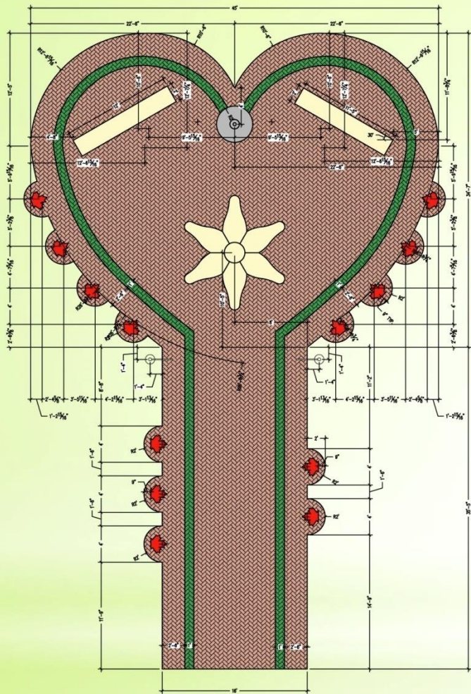
1 PLAN ÉCHELLE: 1/4" = 1'-0"
